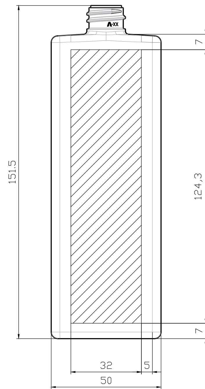
SBM2-120ML 印刷範圍
