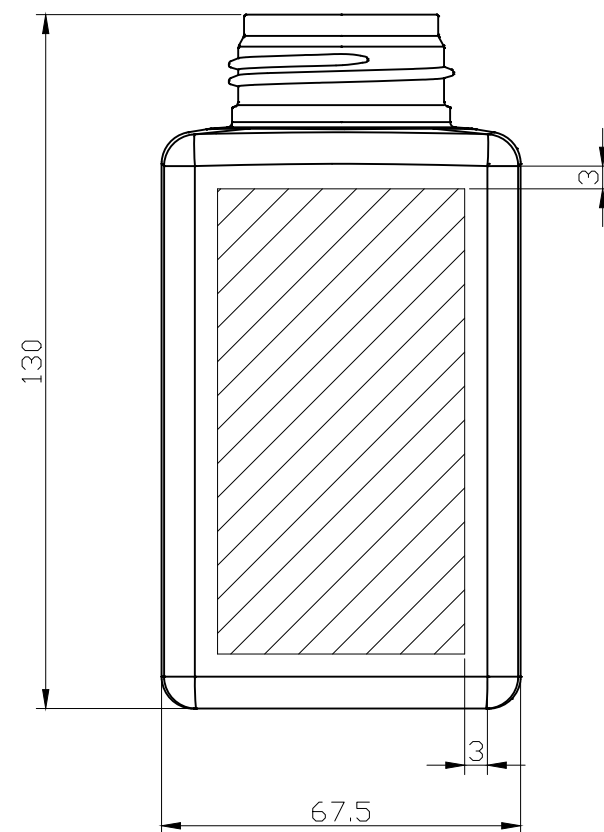
SB07-400ML印刷範圍
