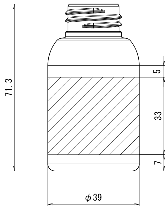
SB08-50C印刷範圍
