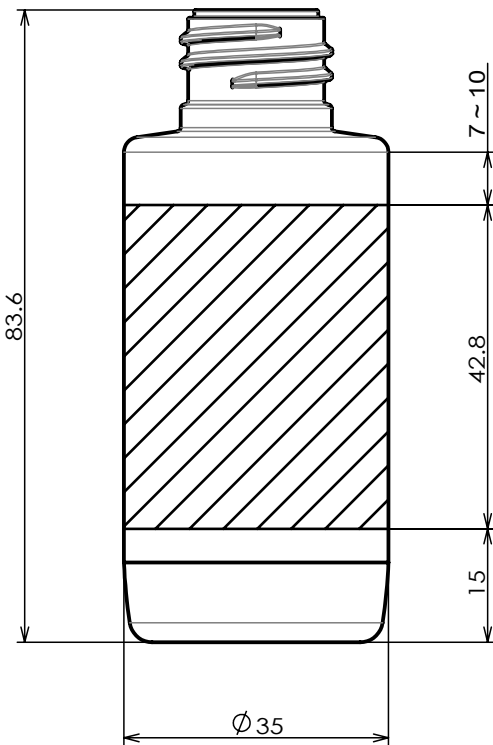
SB05-50C印刷範囲
