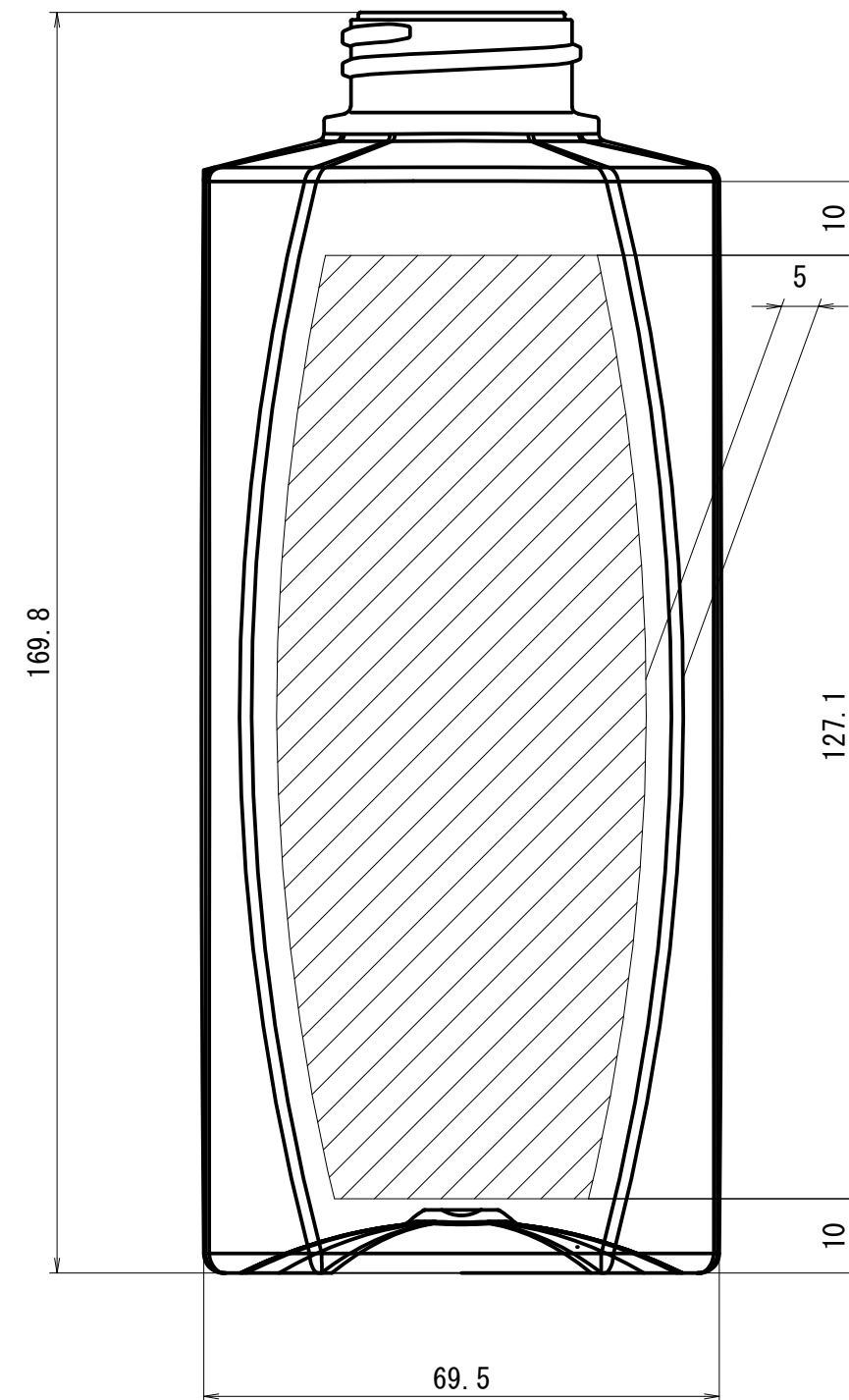
SB04-600ML印刷範圍
