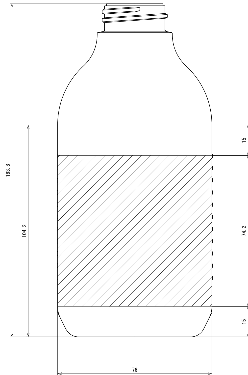
SB04-500UDリブあり印刷範囲
