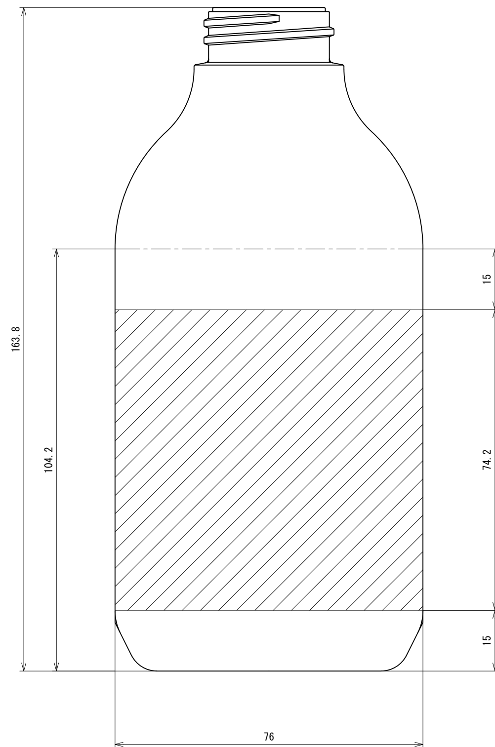
SB04-500UDリブなし印刷範囲
