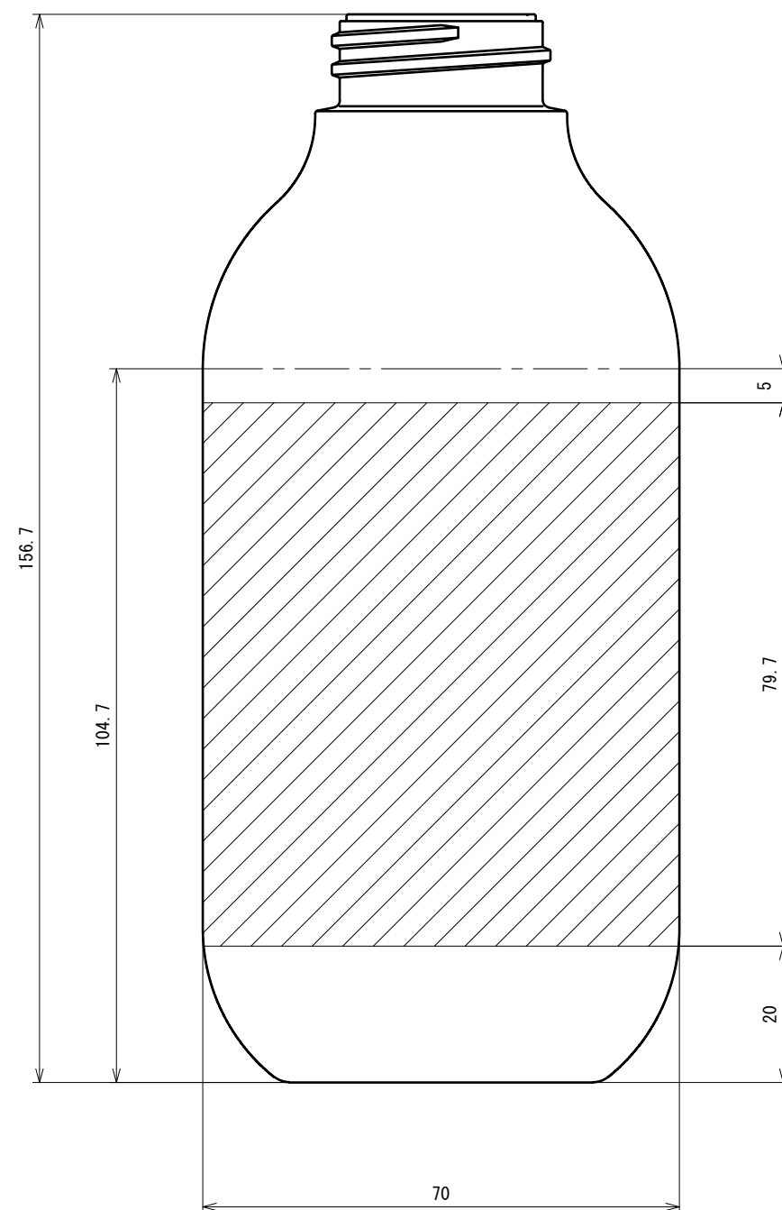
SB04-400UDリブなし印刷範囲
