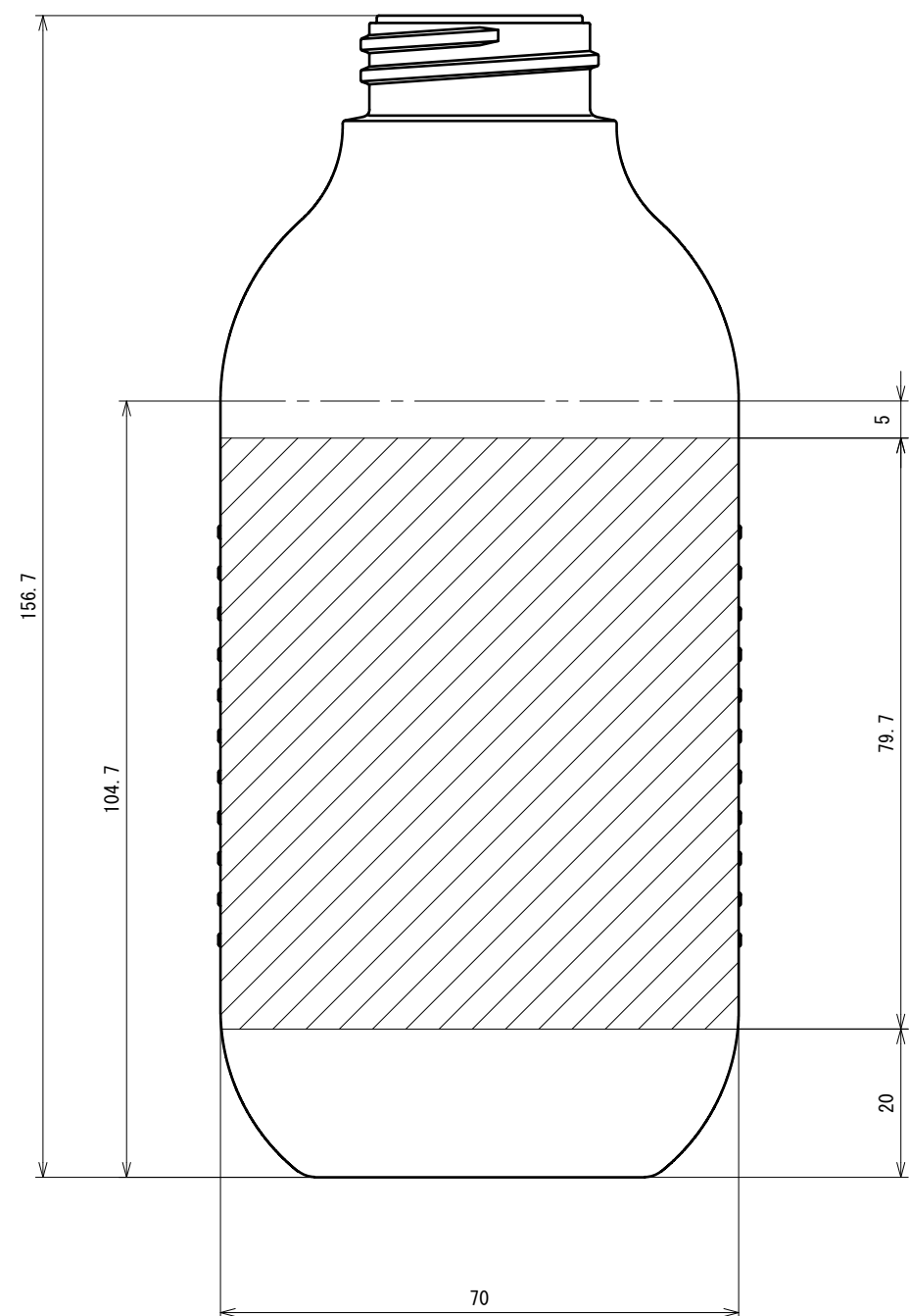
SB04-400UDリブあり印刷範囲
